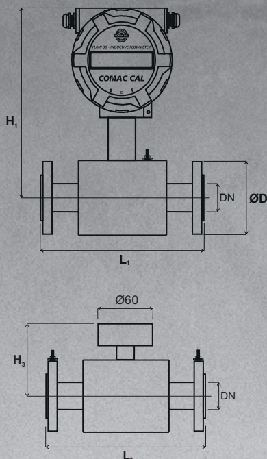
PŘÍRUBOVÉ PŘIPOJENÍ (EN 1092)
